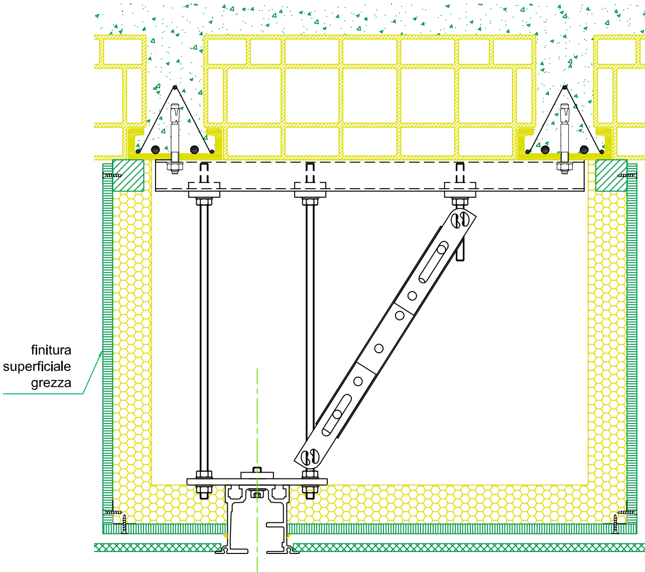
soluzione con controsoffitto
