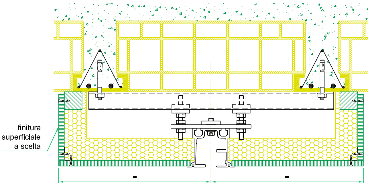
soluzione senza controsoffitto
