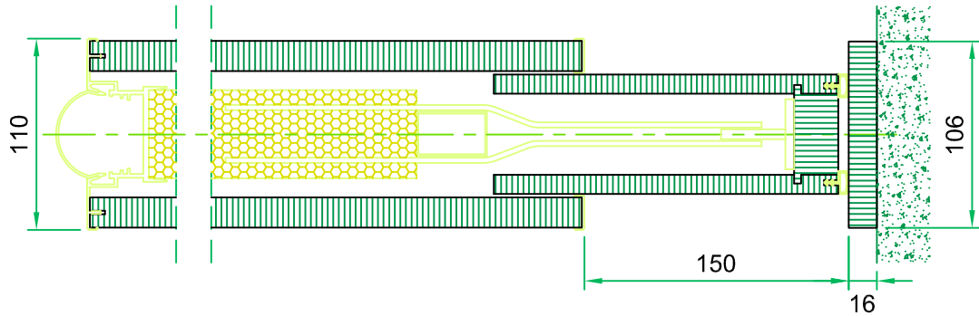
particolare modulo TC bicarrello con profili nascosti su montante di arrivo MA
