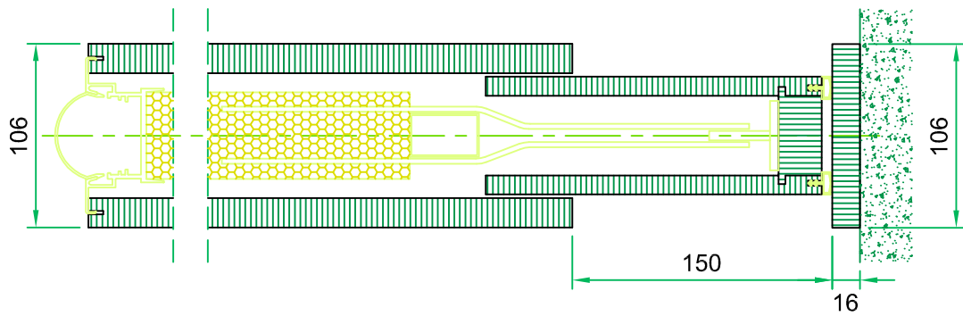
particolare modulo TC monocarrello con profili in vista su montante di arrivo MA
