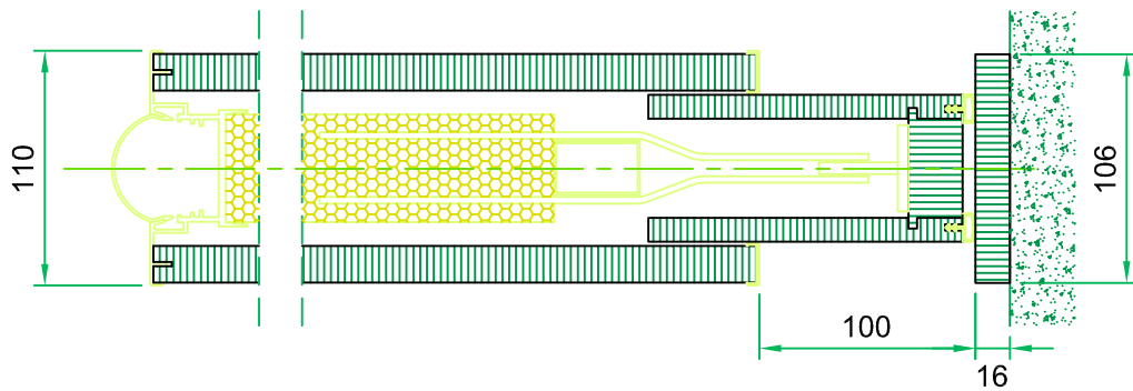
particolare modulo TC monocarrello con profili nascosti su montante di arrivo MA
