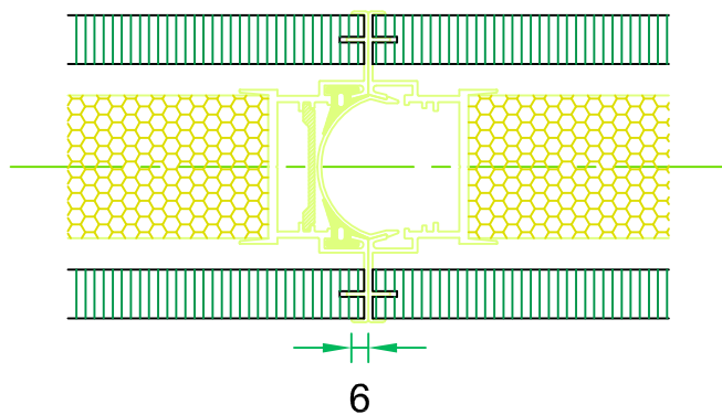
particolare nodo profili in vista
