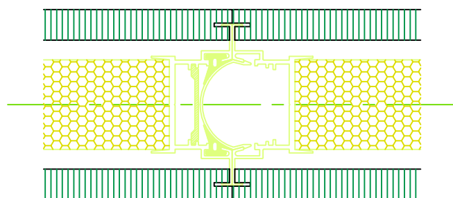
particolare nodo profili nascosti
